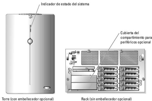
Figura 1-1. Orientación de montaje para torre y rack
