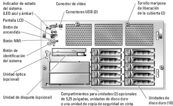
Figura 1-2. Características e indicadores del panel frontal
