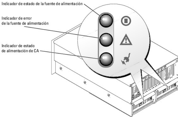
Figura 1-5. Indicadores de fuente de alimentación
